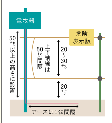
電気柵の設置例(イノシシ対策の場合)
