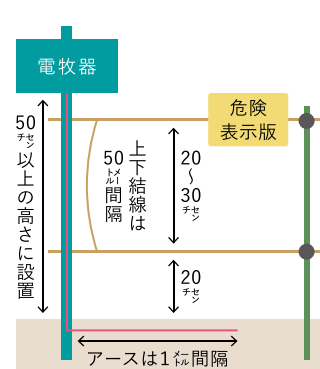
電気柵の設置例(イノシシ対策の場合)
