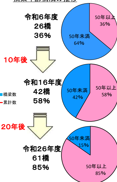
橋梁年齢構成の推移
