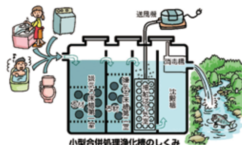
小型合併処理浄化槽のしくみ
