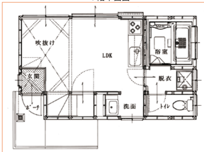
1階平面図
